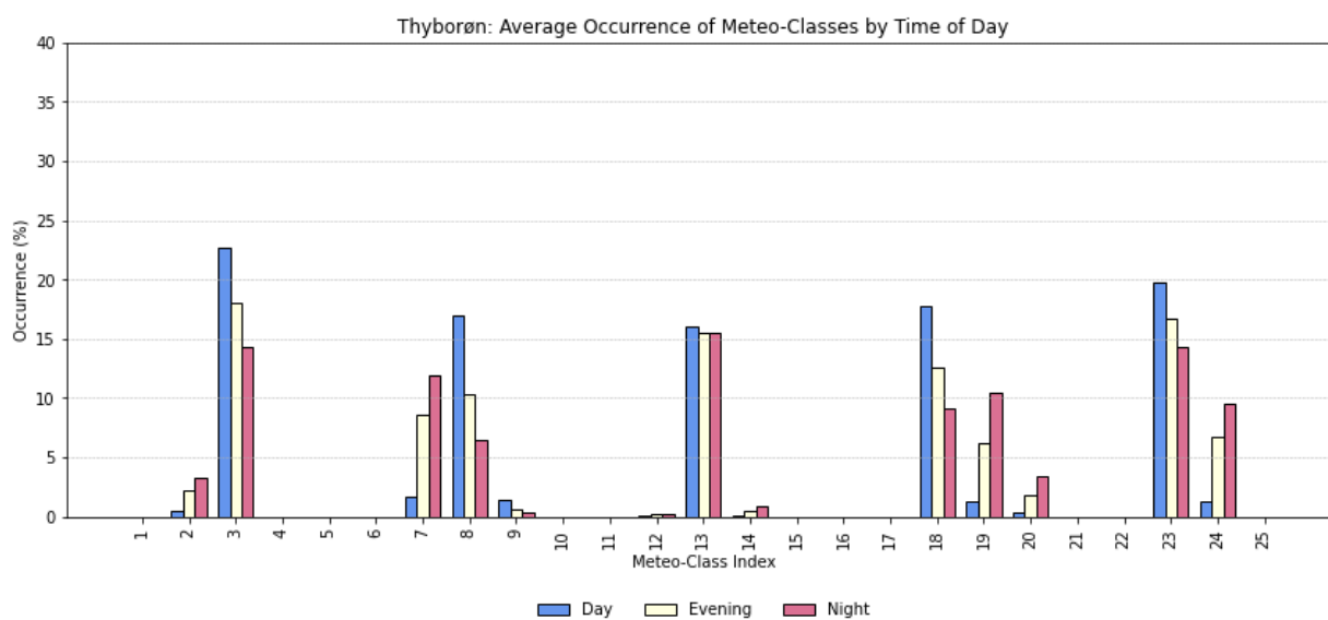
Figur 6 Statistisk fordeling af meteoklasser (middel for alle retninger) udarbejdet for Thyborøn (kyst).
