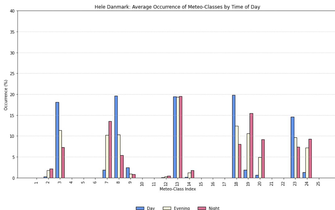
Figur 11 Statistisk fordeling af meteoklasser (middelt for alle retninger) for meteoklasser svarende til et middel af alle de 15 målestationer, der havde tilstrækkeligt med data.
