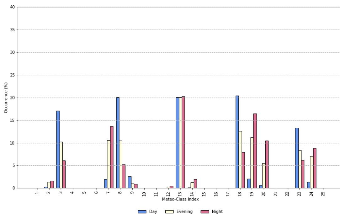
Figur 12 Statistisk fordeling af meteoklasser (middelt for alle retninger) for forslaget til nye meteoklasser svarende til et middel af alle de 12 endelige målestationer.
