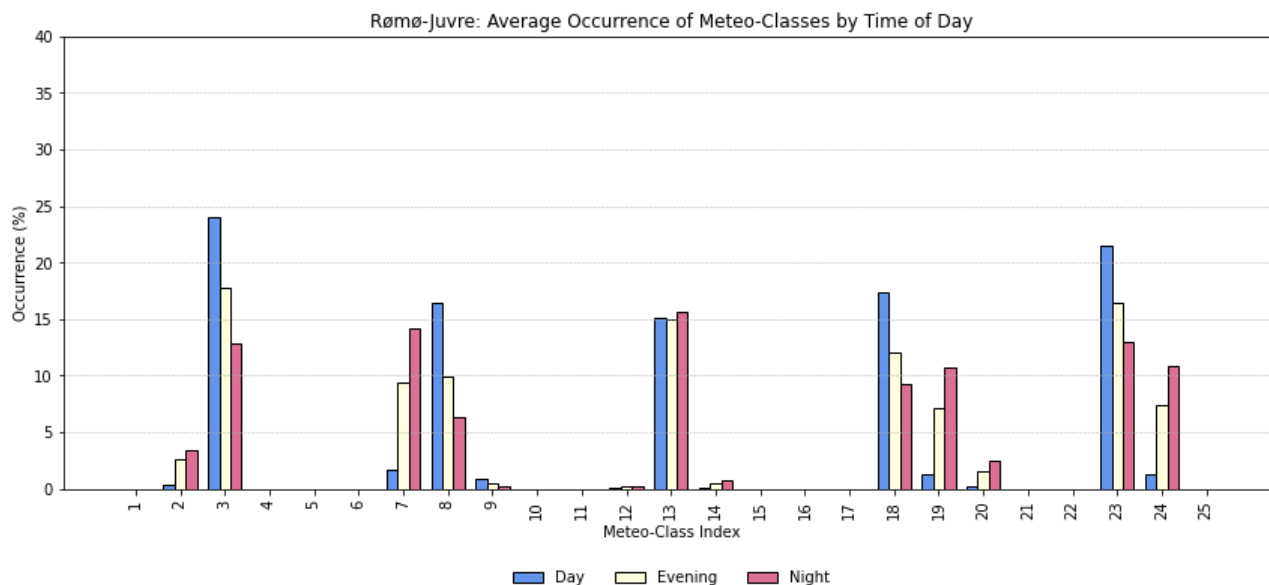
Figur 7 Statistisk fordeling af meteoklasser (middel for alle retninger) udarbejdet for Rømø-Juvre (kyst).
