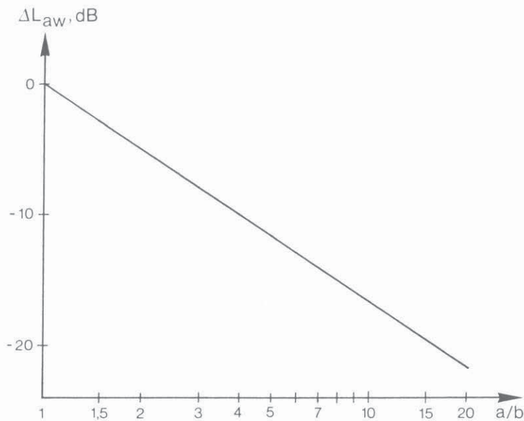
Figur 6 Dæmpning af vægtet vibrationsniveau.
