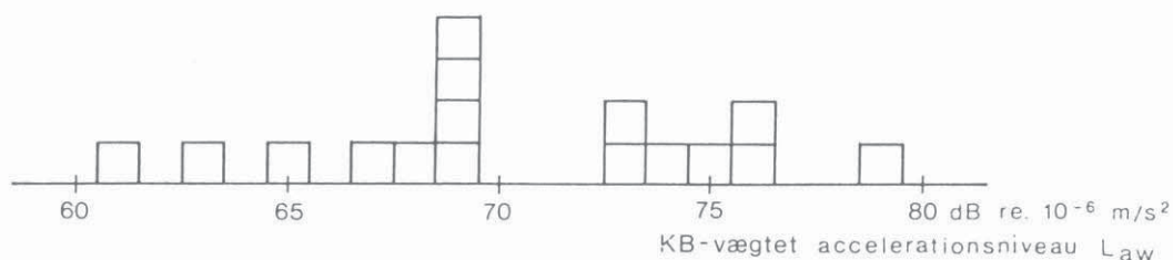
Figur 5 Middelværdi af L_{Aw, maks} ved 8-15 togpassager på hvert af 16 målesteder, målt i jorden i 10-15 m afstand fra sporene.
