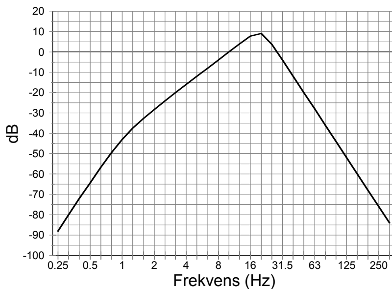
Figur 2 G-filter til måling af infralyd (ISO 7196).
