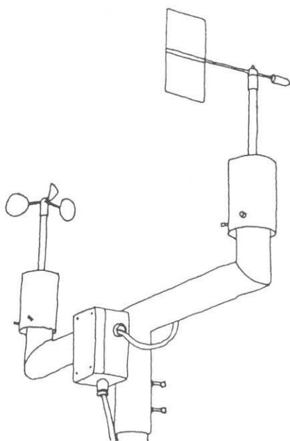
Figur 4a Bom med vindfane og kopanemometer [Vaisala]
