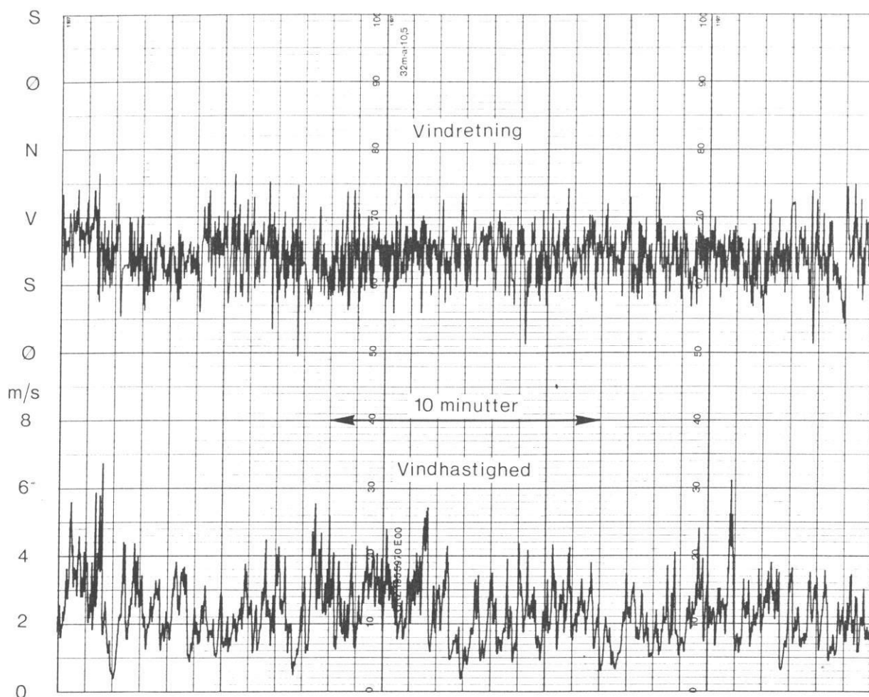
Figur 2 Eksempel på analog registrering af vindhastighed og -retning.
